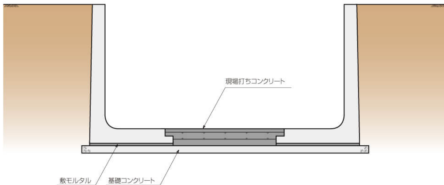
一般図
