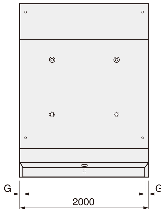
Bタイプ: 砂質土用
