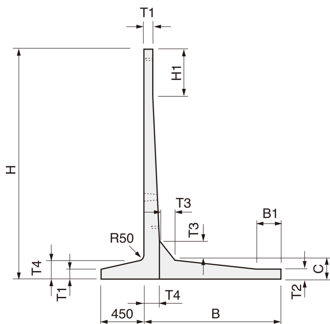
Aタイプ: レキ質土用
