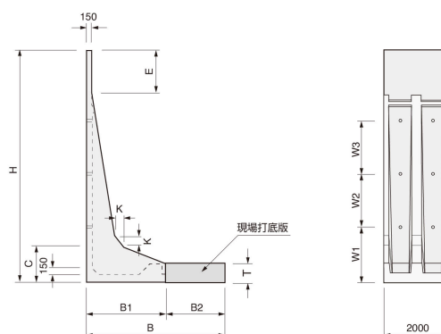
Sタイプ 砂質土
