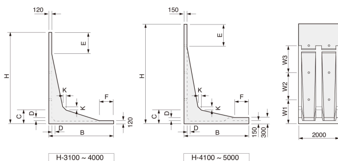
Nタイプ 粘性土
