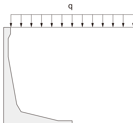
ケース B：載荷重を底版上に載荷する場合
