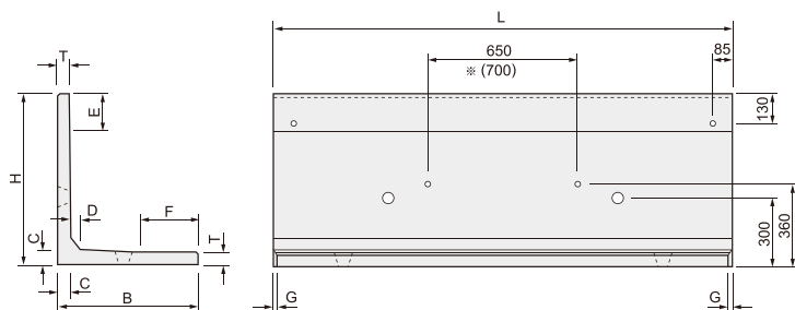
連結用プレート詳細図（F・S・N共通）
