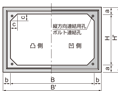
標準タイプ：PC鋼材及びボルトによる縦方向連結型
