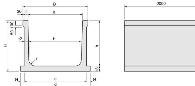
張り出し有りタイプ（浮力対応型）
