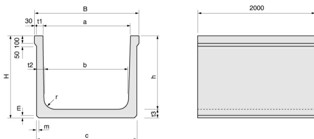
張り出し無しタイプ
