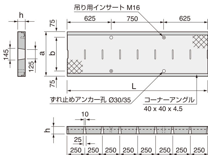
乗入れ横断用 標準部
