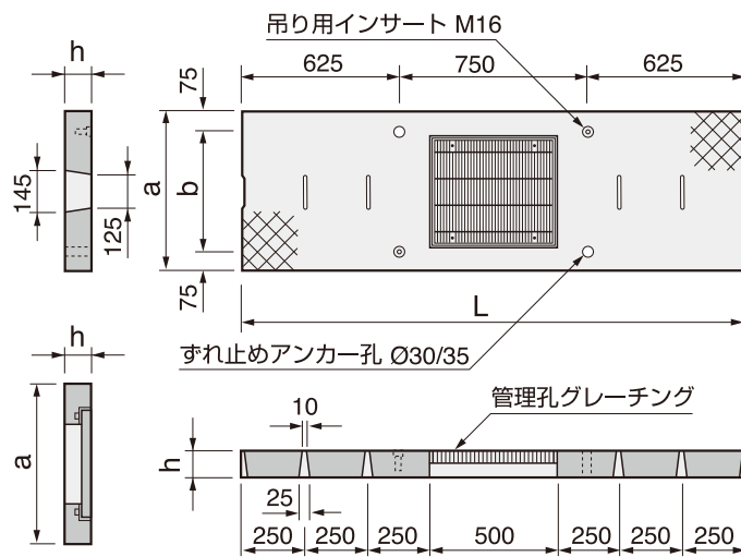
縦断用 管理孔部
